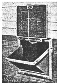
Fig. 182—Iron coal chute
