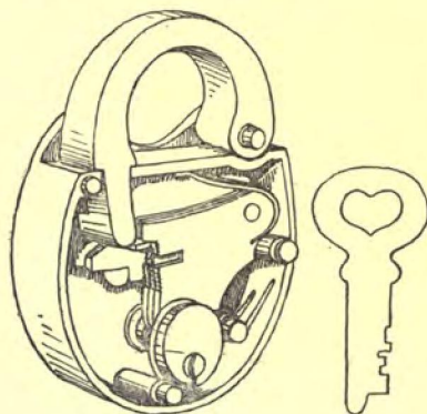
Fig. 352. Padlock. A. E. Dietz.
