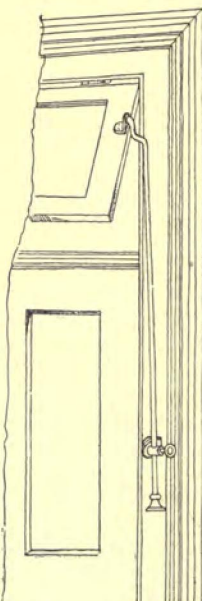
Fig. 275. Excelsior Transom-lifter. Russell & Erwin.
