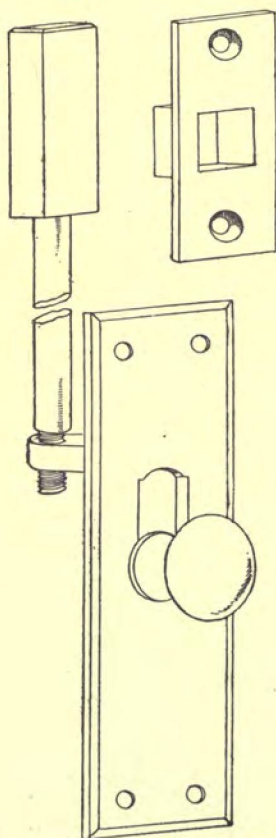
Fig. 43. Mortise Flush Bolt. J. B. Shannon & Co.
