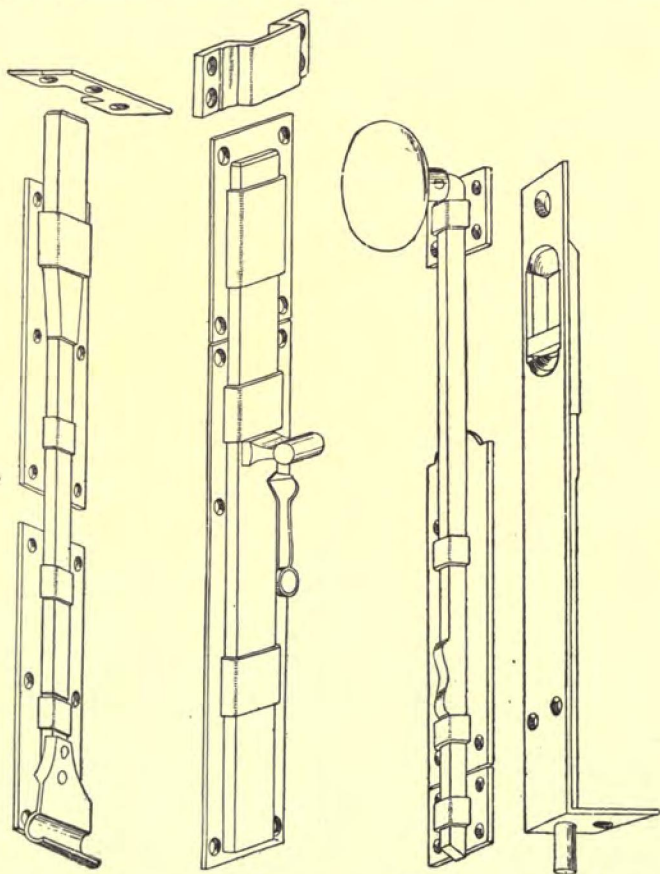
Fig. 38. Flat Tail-Bolt.
