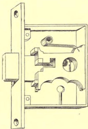
Fig. 298. Mortise Dead-lock. A. G. Newman.
